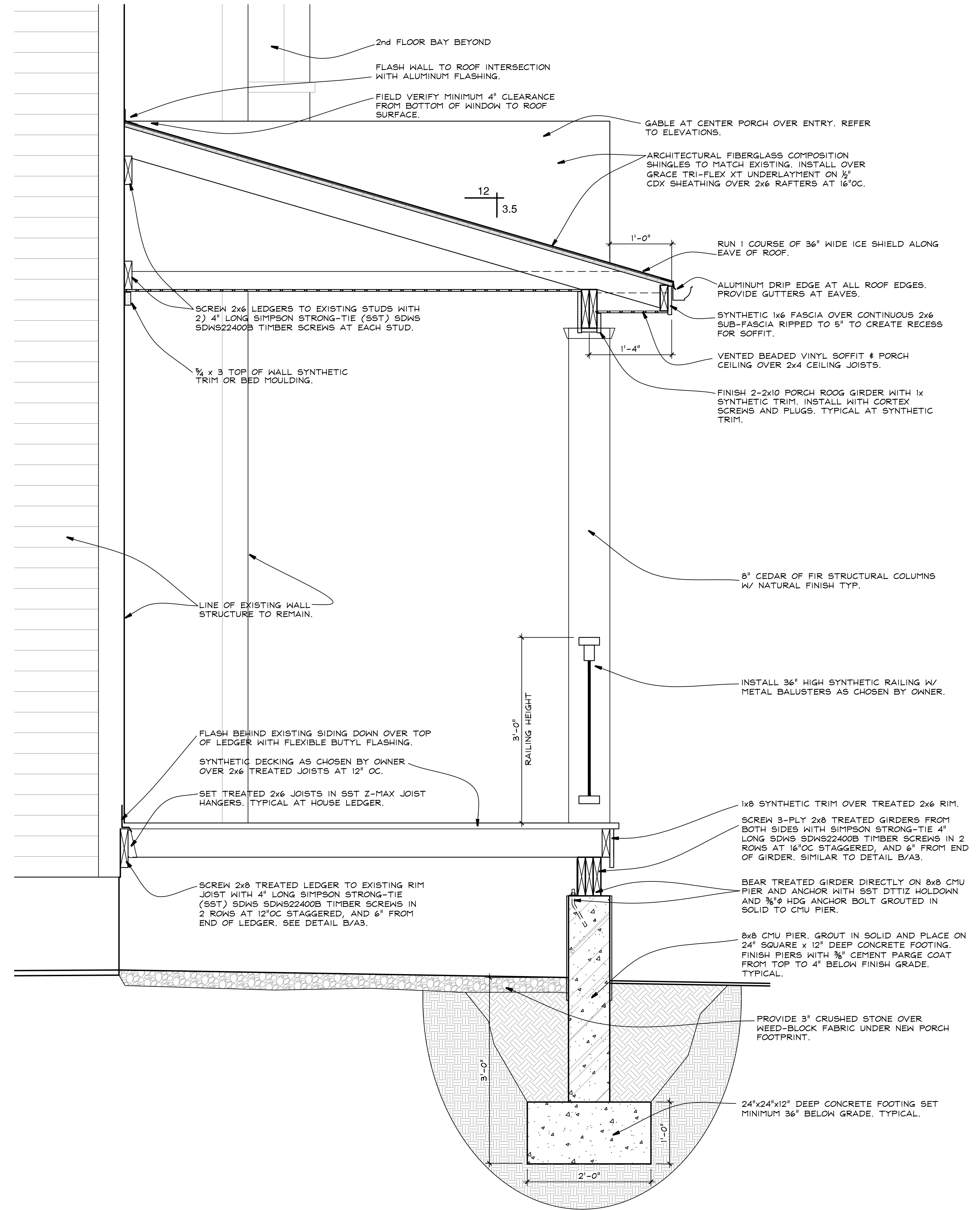
A PORCH SECTION A3 1" = 1 FOOT
